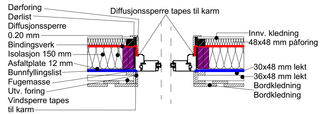
Horizontalschnitt XXX+48 mm
