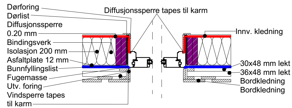
Horizontalsnitt 198 mm
