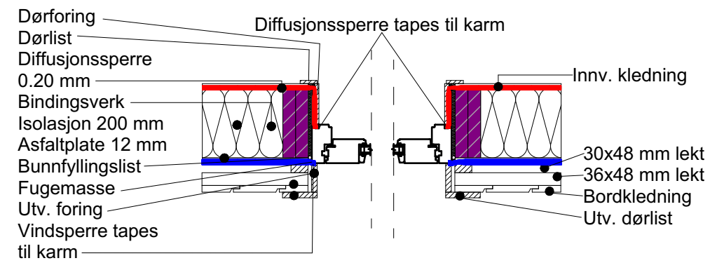
Horizontalsnitt 198 mm
