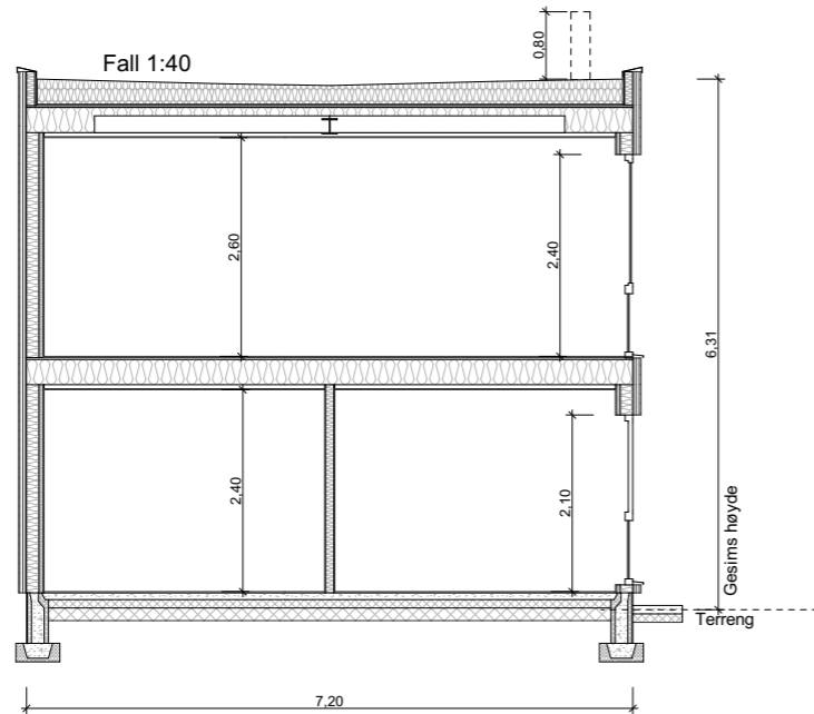
Snitt A 1:100
